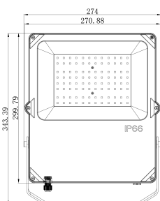
Face avant
