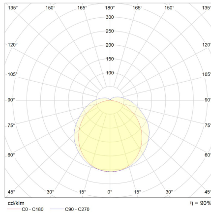
Photométrie ABT07M15I050WF840P
