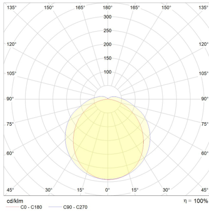
Photométrie ABT07P15I050WF840R
